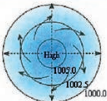
نمای وا چرخند از بالا
