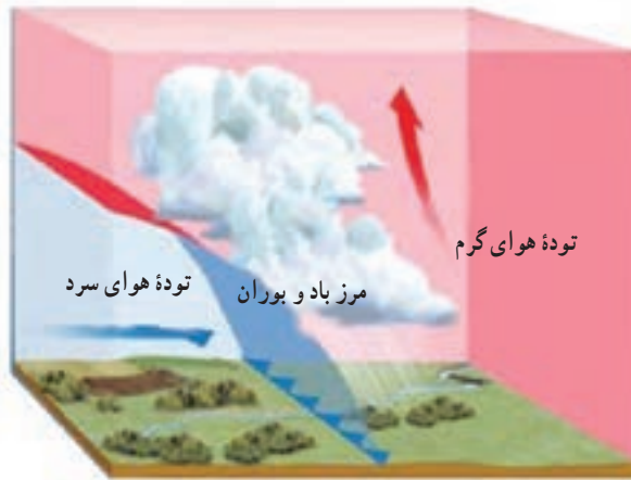
تصویر ۲-۸- جبهه سرد
