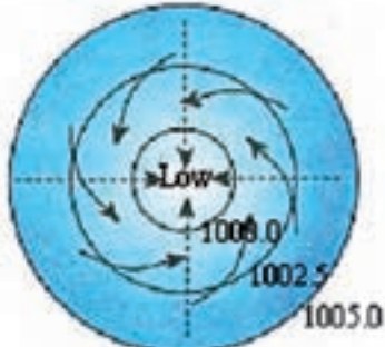
تصویر ۵-۸ - نمای چرخند از پهلو و بالا
