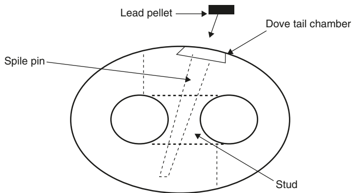
Kenter Lugless joining shackle.
